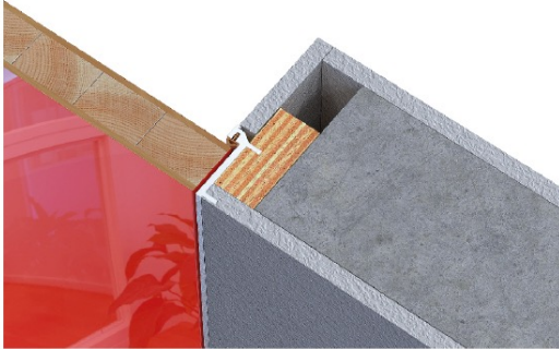
Inswing Hidden Jamb
